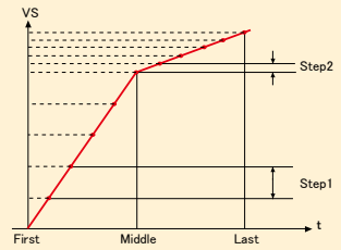
ツーフロー・リニア・スイープ例
