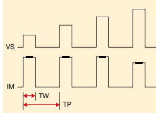
測定波形
