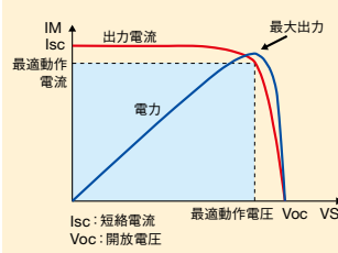
光電圧 - 光電流, 光電圧 - 光電力 特性
