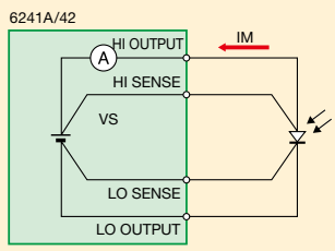
接続図
