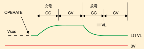
バッテリー充電波形
