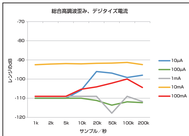
総合高調波歪み (THD) (代表値) 80
