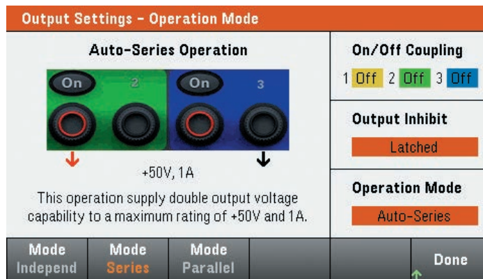
図3. 出力電圧を2倍にする自動直列動作
