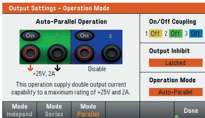
図4. 出力電流を2倍にする自動並列動作
