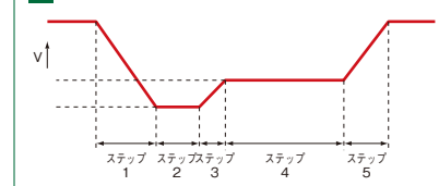
例 電圧変動試験パターン例
