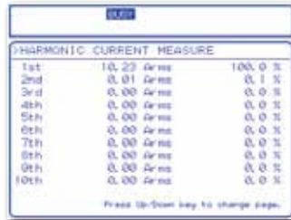
▲出力高調波電流計測
