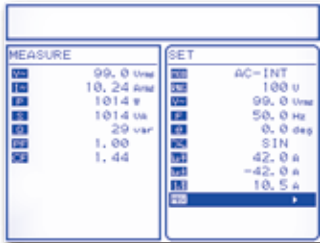
▲計測結果と設定値
