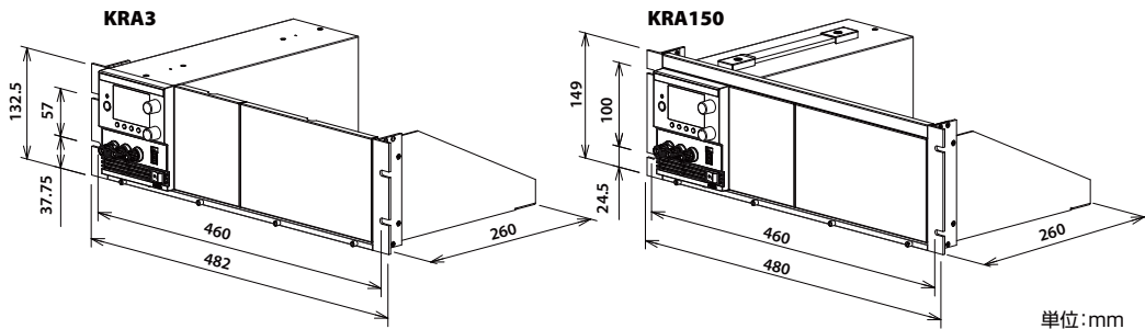
単位:mm
