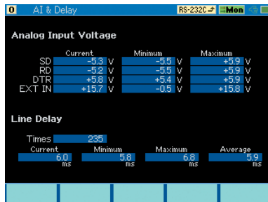
【アナログ&デレータイム測定表示例】
