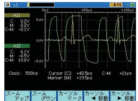
【アナログ波形解析表示例】
