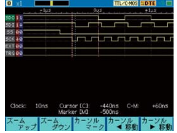
【SPIのデジタル波形測定例】
