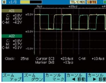
【I 2 Cのアナログ波形測定例】
