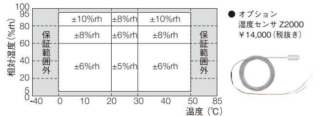
湿度センサ Z2000 使用時確度表
