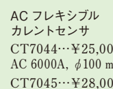
AC フレキシブル カレントセンサ CT7044... ¥25,000 AC 6000A, φ100 mm CT7045... ¥28,000 AC 6000A, φ180 mm CT7046... ¥30,000 AC 6000A, φ254 mm
