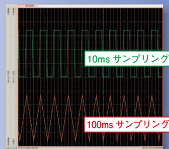
5Hz のパルス波形を 10ms と 100ms でサンプリング
