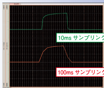
負荷が急変する波形を 10ms と 100ms でサンプリング
