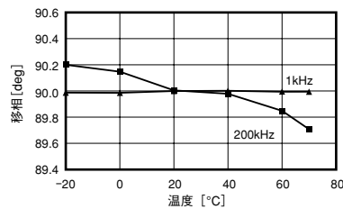
90° 移相誤差 - 温度特性
