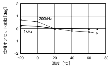
位相オフセット - 温度特性
