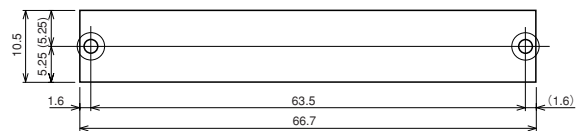
最大外形寸法
