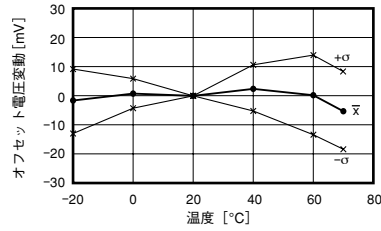
オフセット電圧 - 温度特性
