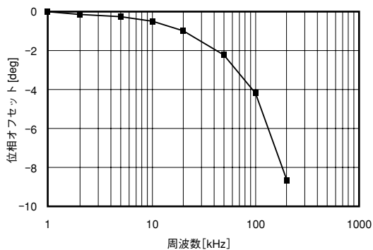
位相オフセット
