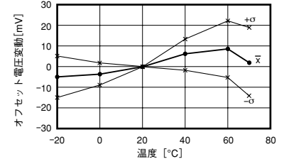
オフセット電圧 - 温度特性
