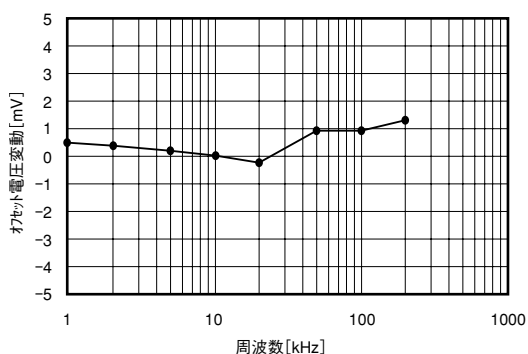
オフセット電圧変動 10kHz基準 利得10倍
