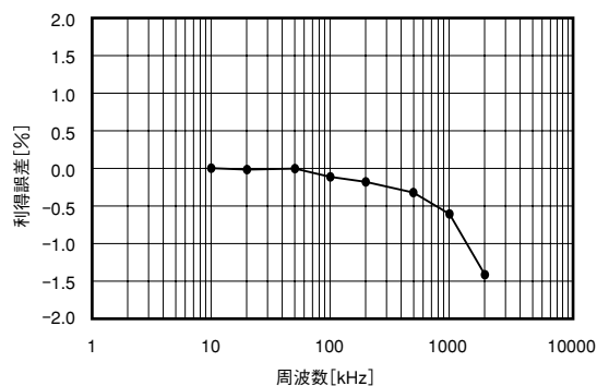
利得変動 10kHz基準 利得10倍
