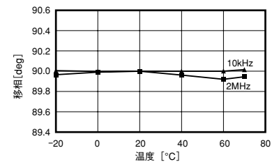
90° 移相誤差 - 温度特性
