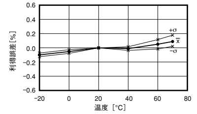
利得誤差 - 温度特性
