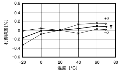
利得誤差 - 温度特性
