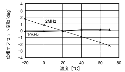
位相オフセット - 温度特性
