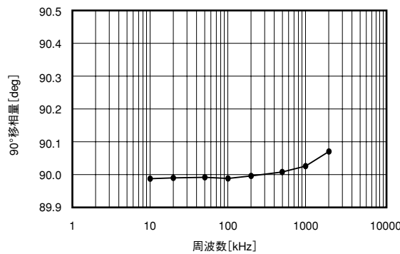
90° 移相量変動
