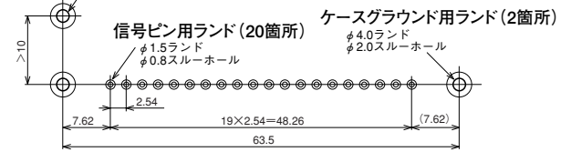
パターン寸法図
