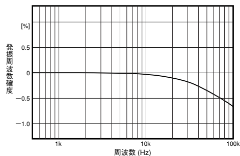
発振周波数確度 (CG-402R2)
