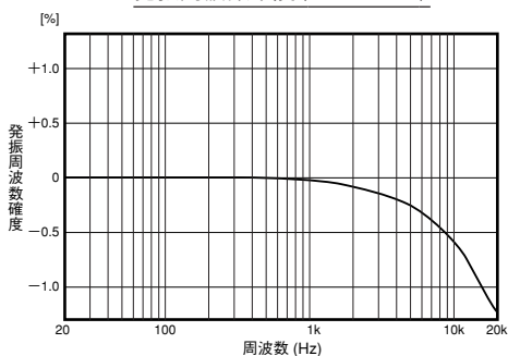
発振周波数確度 (CG-402R1)
