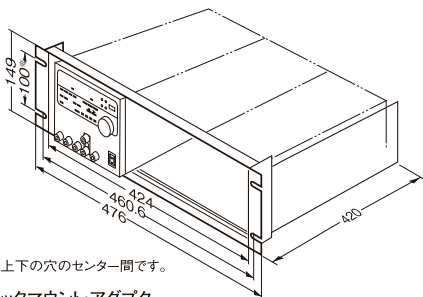
※上下の穴のセンター間です。 ラックマウント・アダプタ RM-608E (EIA)
