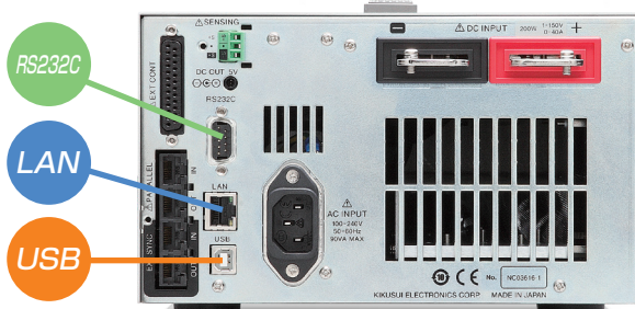
リアパネル
