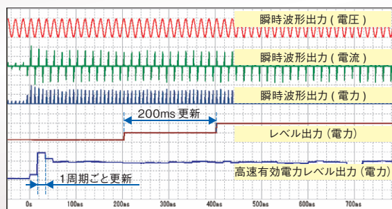
ファンモータ起動時の D/A 出力波形
