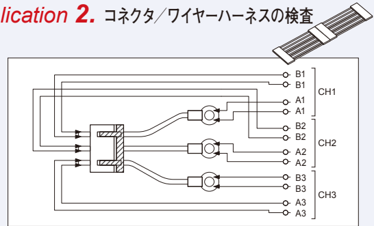
マルチプレクサユニット Z3003 (オプション)
