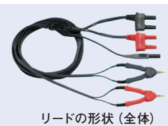
リードの形状 (全体)
