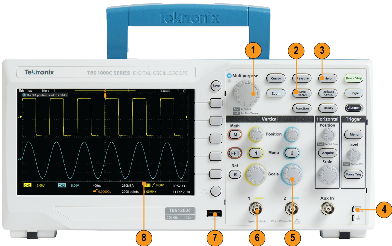
図1: TBS1000C シリーズの前面パネル
