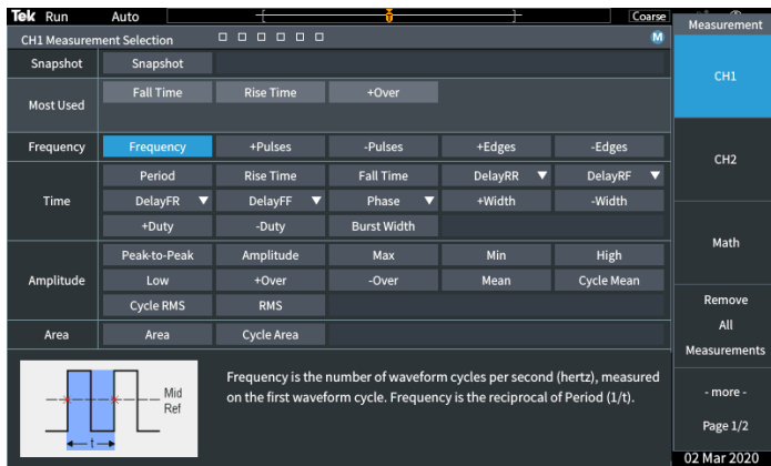
図4: すべての測定項目が1つの画面に表示されるため、簡単に選択できる
