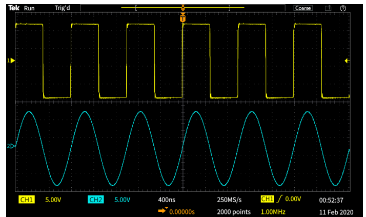
図3: ズーム・モードでは、レコード長全体がディスプレイの上部に表示され、下部には詳細な拡大図が表示される
