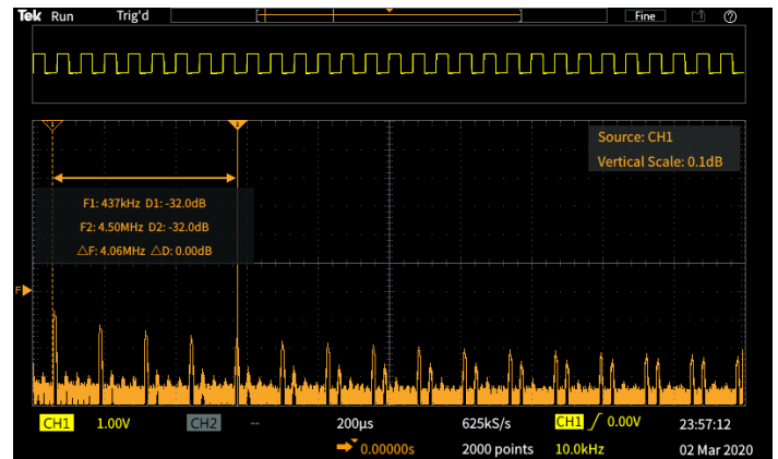
図6: 時間領域波形はFFT波形スペクトラムの上に表示可能
