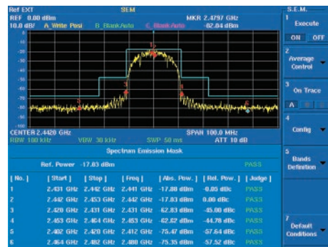
無線LAN S.E.M.測定例
