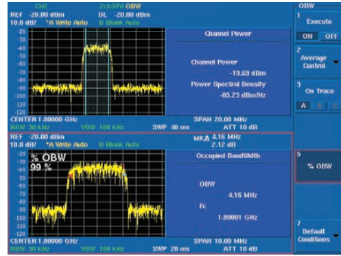
チャンネル・パワーとOBWの同時測定
