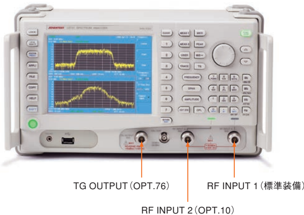
フロント・パネル・コネクタ配置(U3741の場合)
