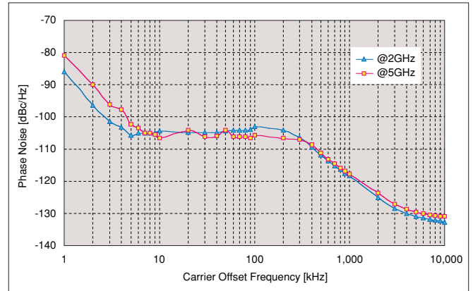
位相雑音特性グラフ(代表値)
