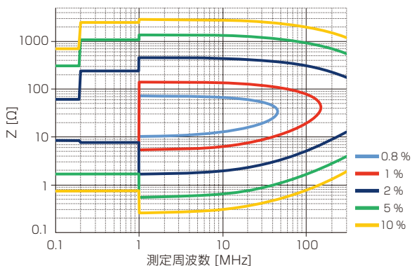
IM7580A / IM7581 (-7dBm ~ +7dBm, SLOW2 の時)
