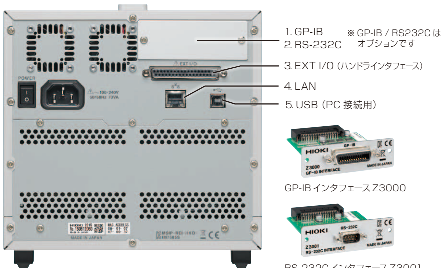
IM7585 本体背面 (インタフェースは4モデル共通)
