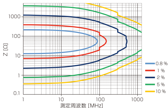
IM7583 / IM7585 (+1dBm, SLOW2 の時)
