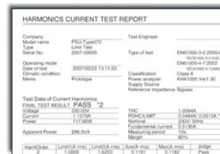
▲テストレポート例 (高調波適合試験)
