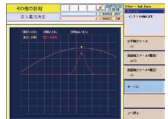
▲ 突入電流測定画面（KHA1000）
