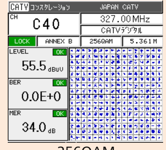
256QAM コンスタレーション表示
