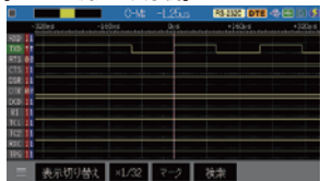
【ロジアナ測定の表示例】
