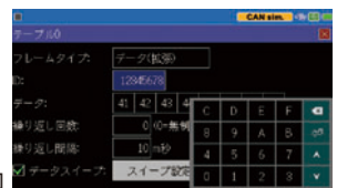
[CANシミュレーションデータ編集画面]
