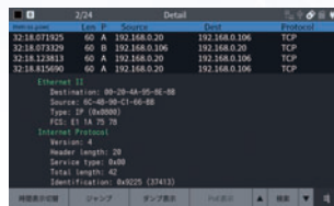
[ LANパケット計測データ表示画面 ]
