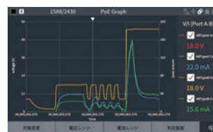
[ PoE計測値 グラフ表示 ]
