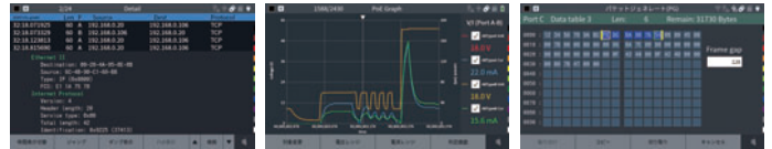
[ LAN/パケット計測データ表示画面 ] [ PoE計測値 グラフ表示 ] [ PGデータ編集 ]
