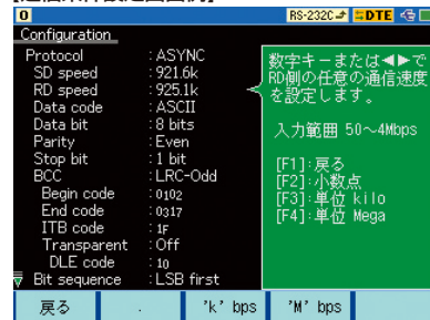
【通信条件設定画面例】
