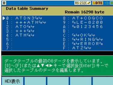
【データテーブル設定例】
