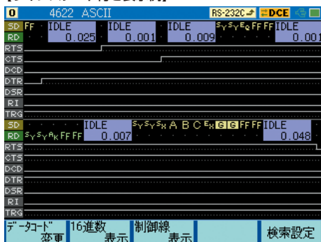
【ラインスタート付き表示例】
