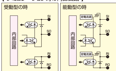
【シミュレーション時の内部回路】
