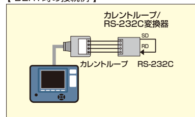
【BERT時の接続例】
