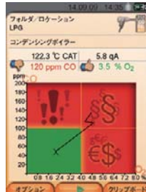
燃焼状態が一目でわかる 排ガスマトリックス
